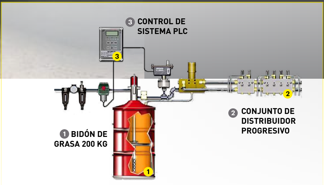
ENGRASE AUTOMATIZADO DESDE BIDÓN DE 200KG
